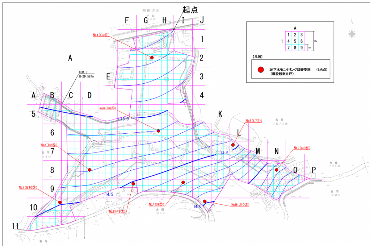
地下水位等高線図 (2021年4月)
