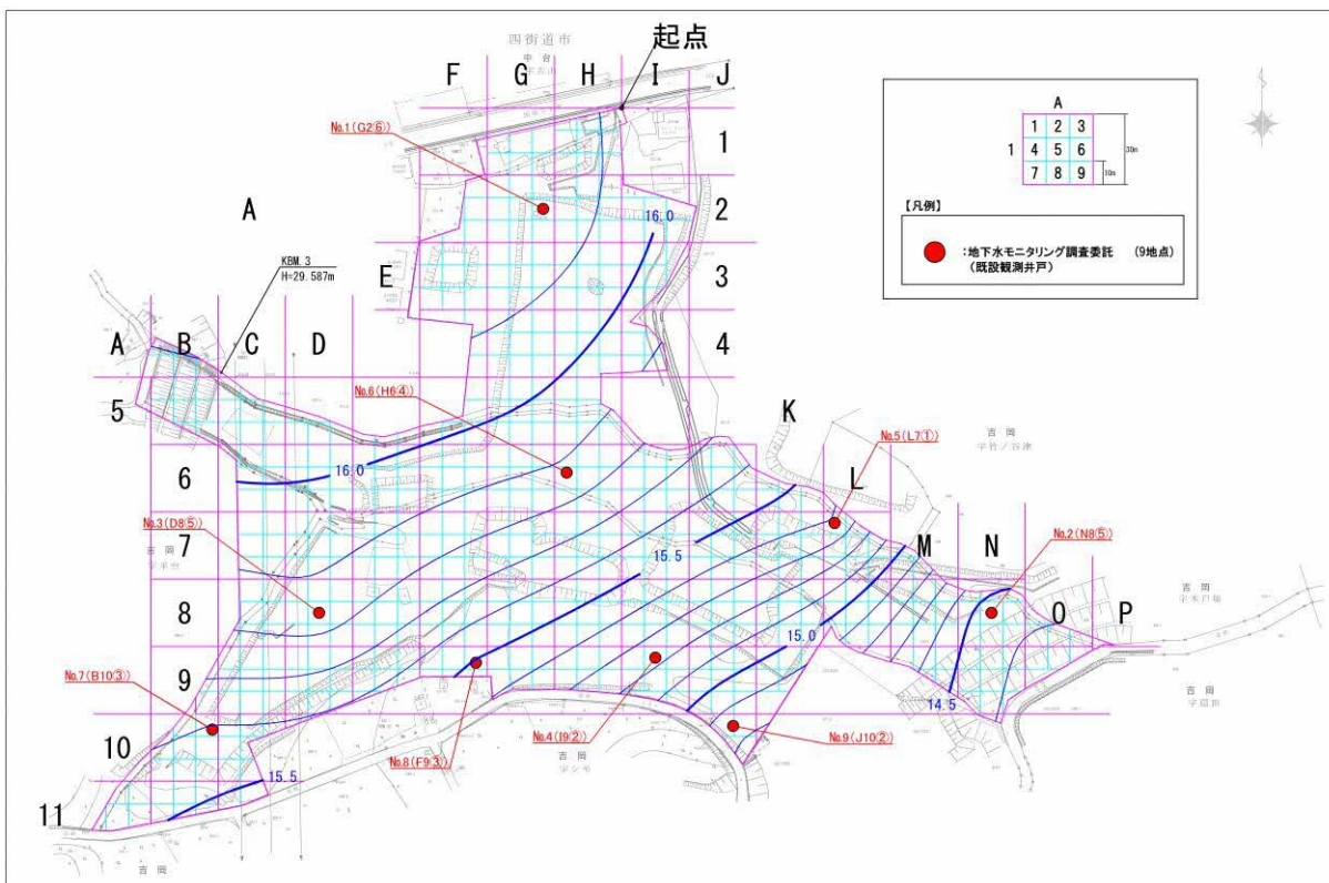
地下水位等高線図 (2021年10月)
