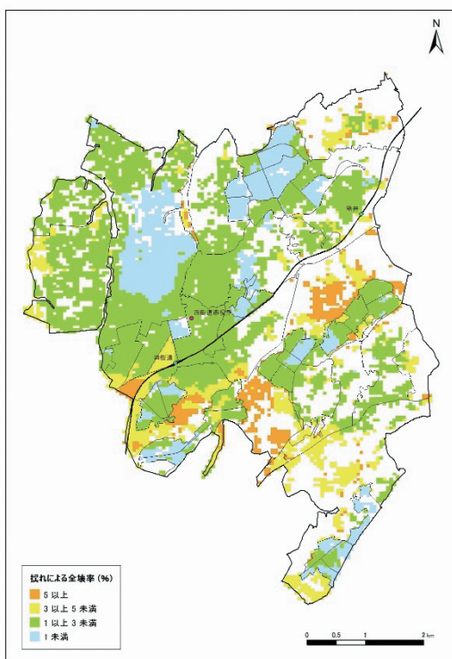
図9 東京湾北部地震(M7.3)の揺れによる建物の全壊率
