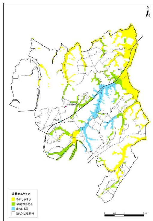
図10 東京湾北部地震(M7.3)による液状化危険度分布
